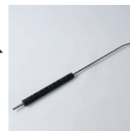
HD-Lanze 100 cm Edelstahl, 15° abgewinkelt Lance haute pression 100 cm en acier inox, coudé Art. Nr. / N° article KCU999352 Ergonomisch geformt, mit Schnellverschluss Forme ergonomique, avec raccord rapide
