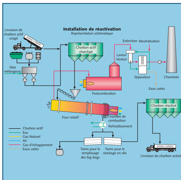
Schéma d'une installation de réactivation de Donau Carbon
