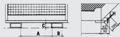
Einfahrtaschen-Innenmaße (mm)
