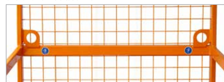
Anschlagpunkte für PSA (Persönliche Schutzausrüstung)
