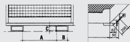
Einfahrbügel-Innenmaße (mm)
