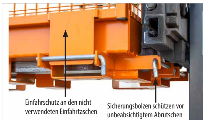
Sicherung der abklappbaren Schutzgitter Kurzanleitung
