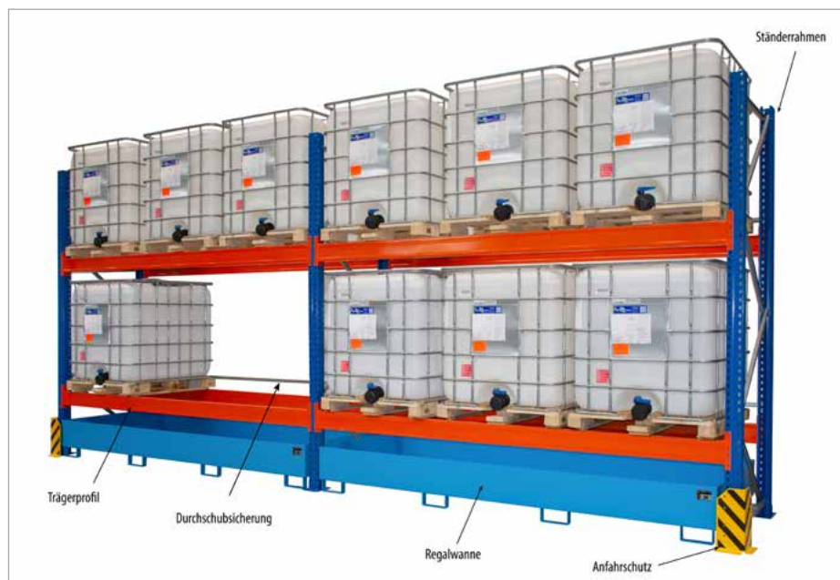
Grundregal UR-G 3300 und Anbauregal UR-A 3300 mit 2x RW 3300-3, Anfahrschutz (Zubehör)
