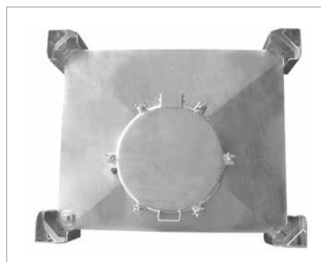
Versetzter Domdeckel
