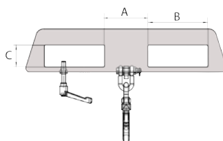
Einfahrtaschen-Innenmaße (Skizze Typ LH-II)
