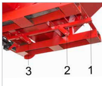
... 3 automatische Entriegelungspunkte
