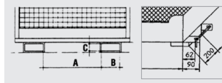
Einfahrtaschen-Innenmaße (mm)
