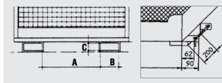
Einfahrtaschen-Innenmaße (mm)
